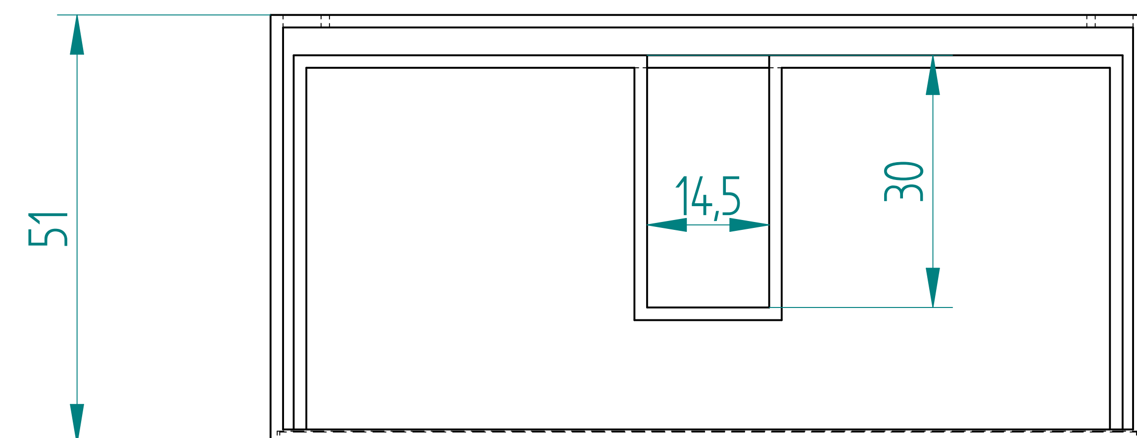
TOP
